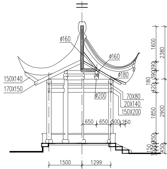
1-1剖面图 1:50
