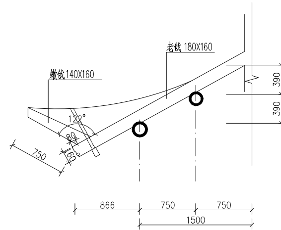
餞角大样 1:25
