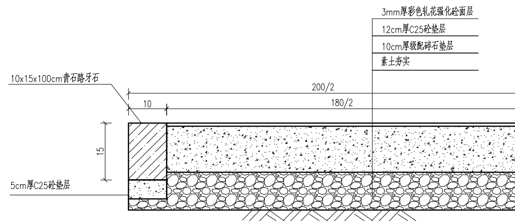
游步道硬化断面图 1:10
