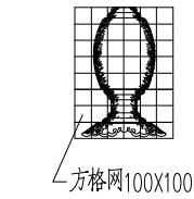
宝顶大样 1:25
