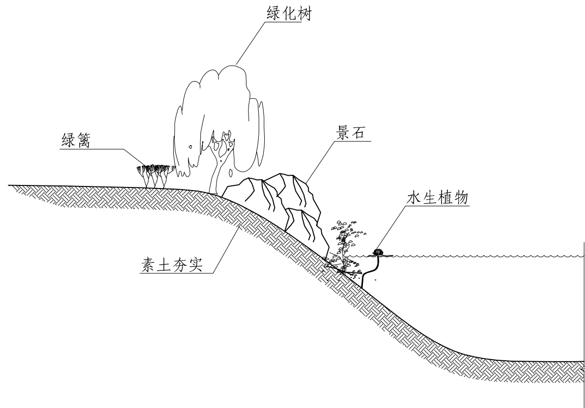
景石安置示意图
