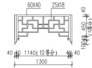
挂落大样 1:25
