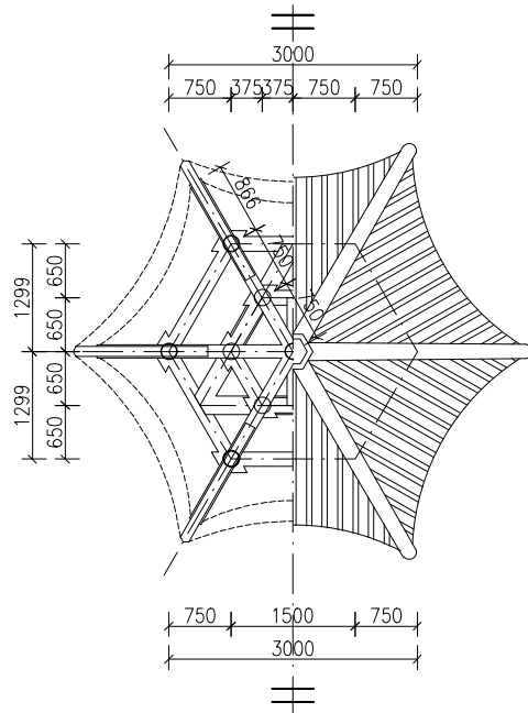
屋架、屋面平面 1:50
