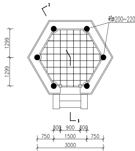
六角亭平面图 1:50
