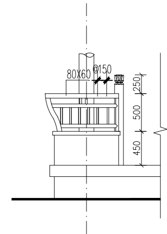
吴王靠大样 1:25
