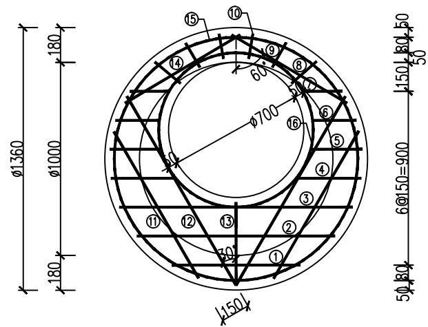
GB-1 配筋图 1:50 盖板厚120mm
