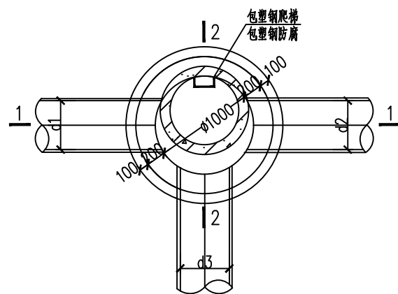
φ1000检查井平面图 1:50
