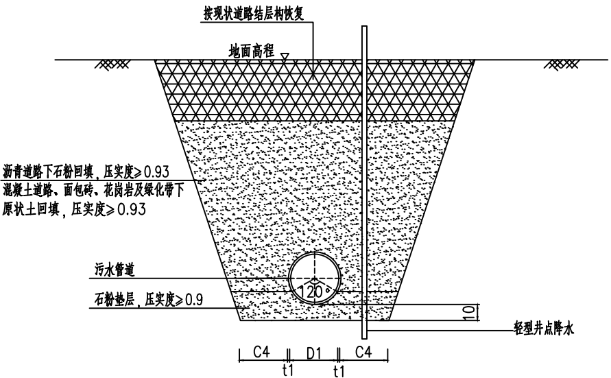
污水管道开挖断面图 1:30
