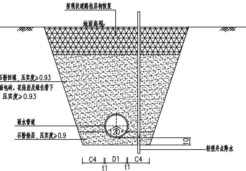
雨水管道开挖断面图 1:30
