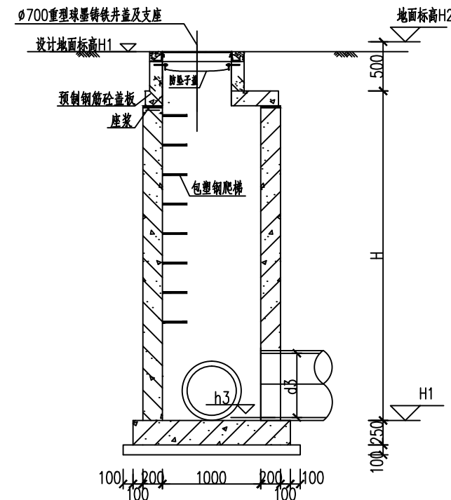
2-2 1:50 (剖面图)
