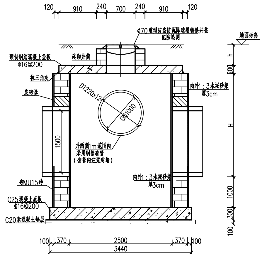
交叉井 1:50 (2.0m×2.5m)
