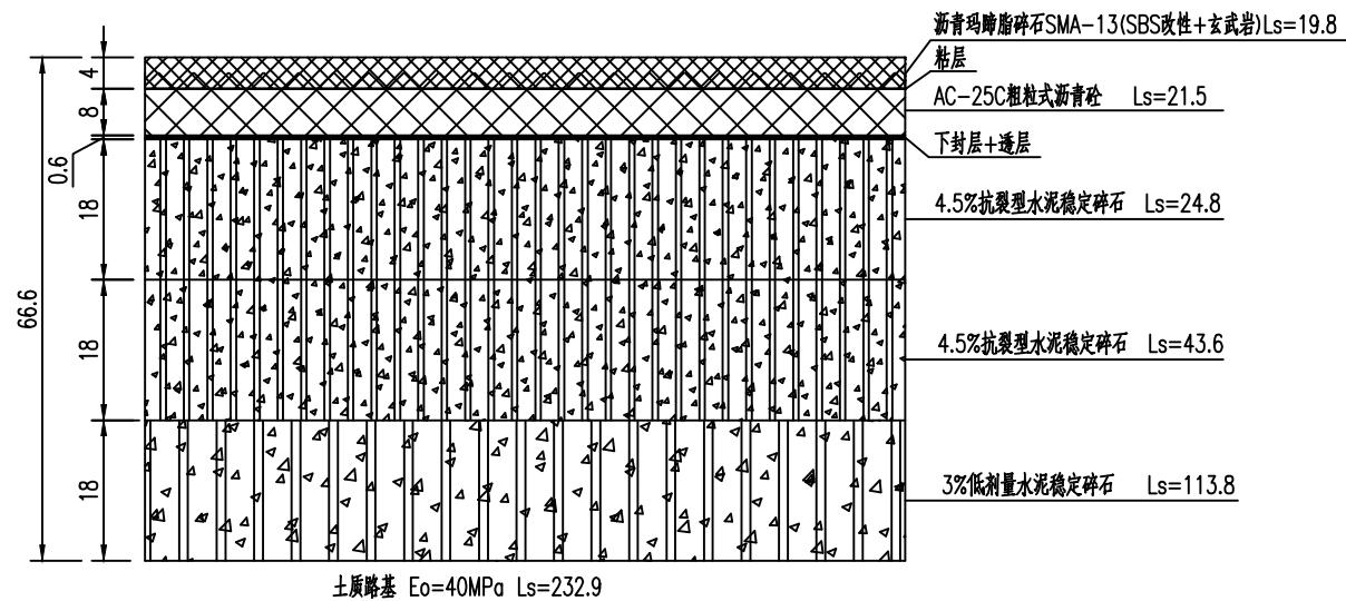
沥青路面结构图
