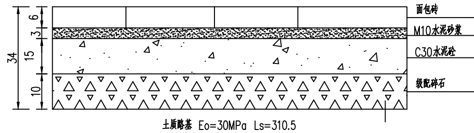
面包砖路面结构图
