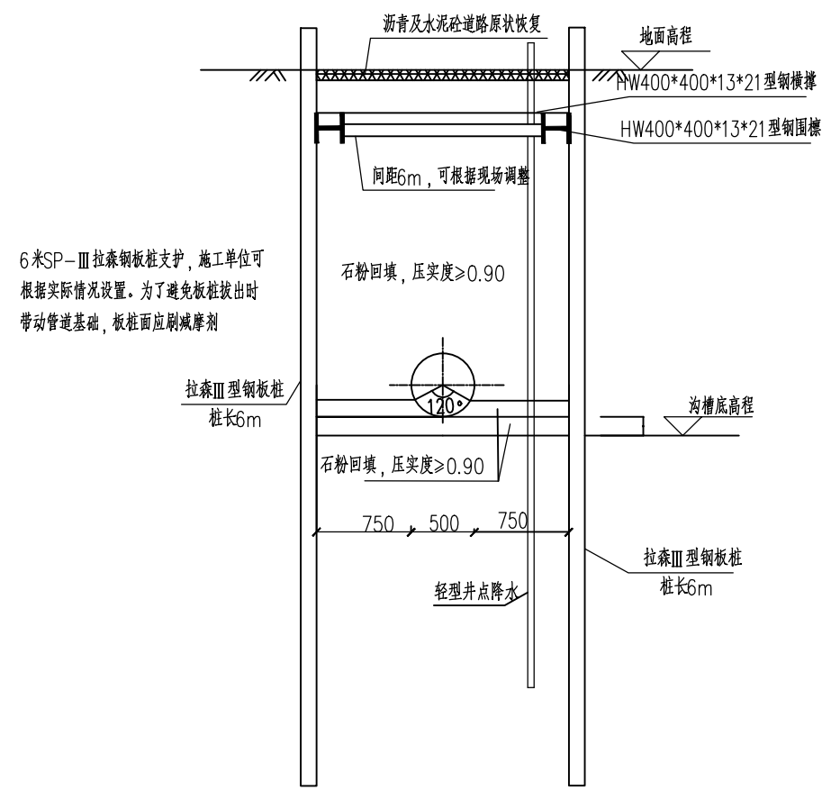
DN500污水管道沟槽开挖回填断面图 1:50 位于沥青道路下
