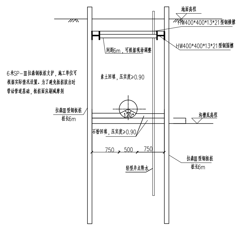
DN500污水管道沟槽开挖回填断面图 1:50 位于绿化带下
