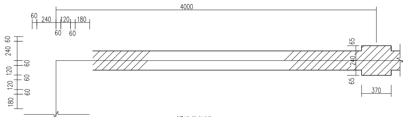
围墙结构图
