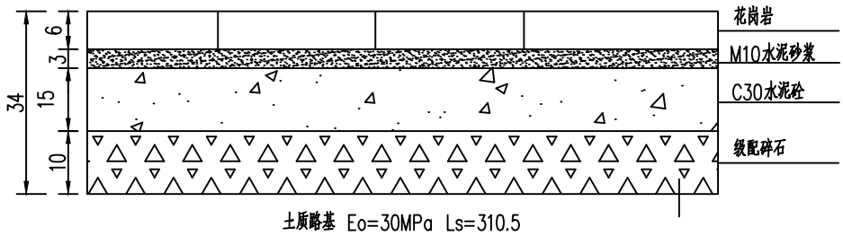
花岗岩路面结构图
