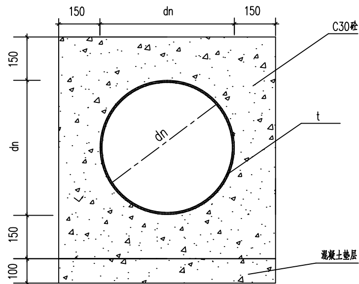
管道包封大样图
