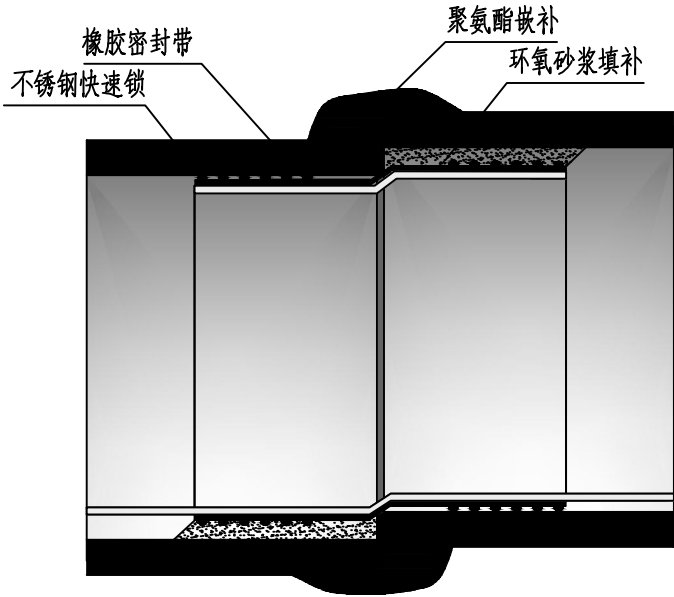
环氧砂浆填补加不锈钢快速锁修补大样图 1:10
