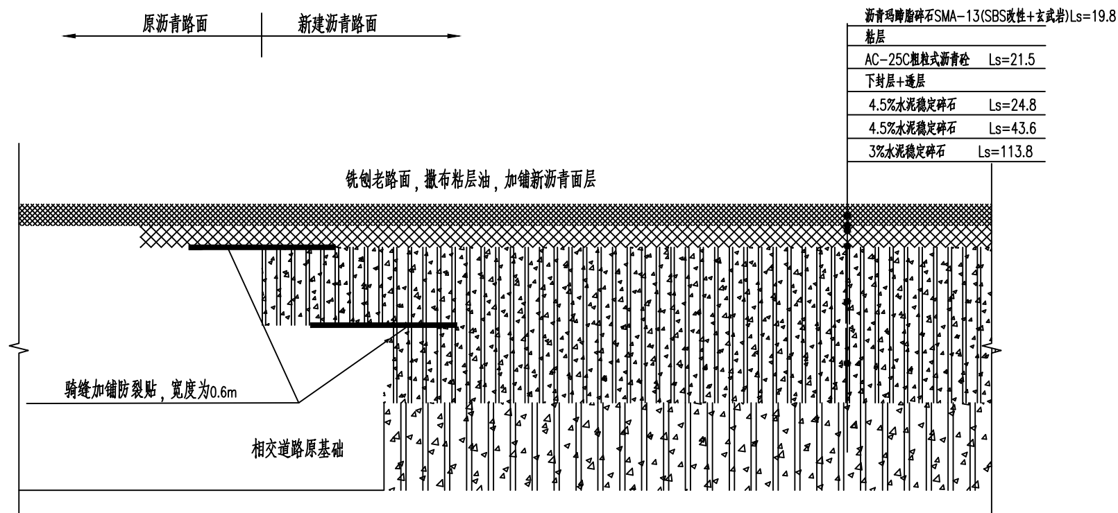
新建沥青路面与原沥青路面搭接处理图
