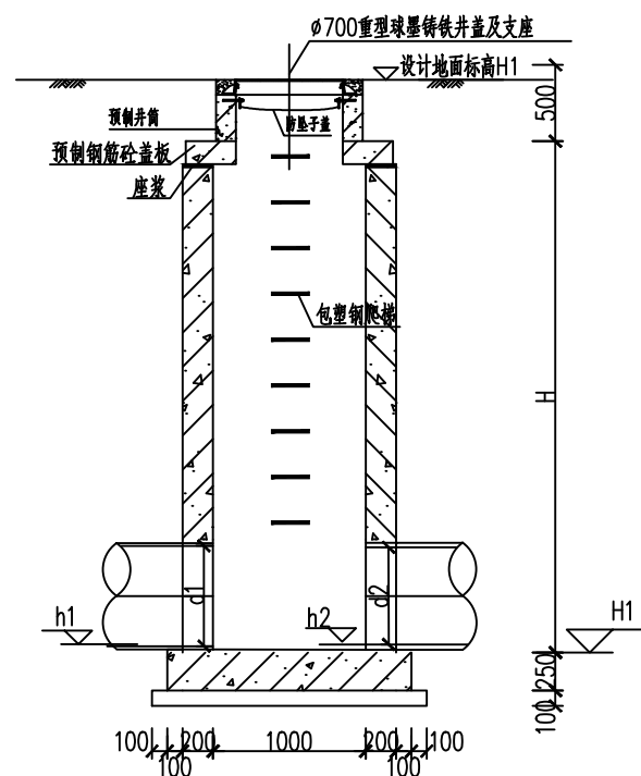
1-1 1:50 (剖面图)
